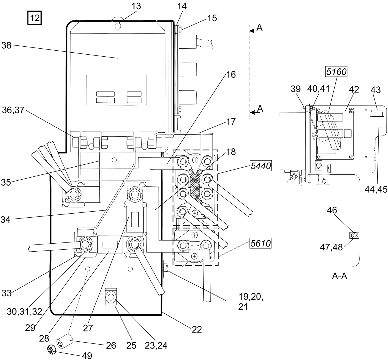
5710-00027 Drive/multi-function PCBs [2003-04-30] Elektronikkort åkning/kombination; Elektronikkarten Fahren/Kombination; Cartes électroniques déplacement/combinaison;
